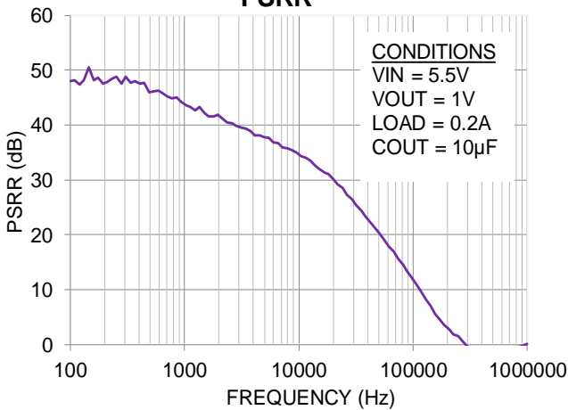
PSRR
